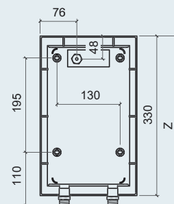
Компактний розмір, патрубки під'єднання знизу
